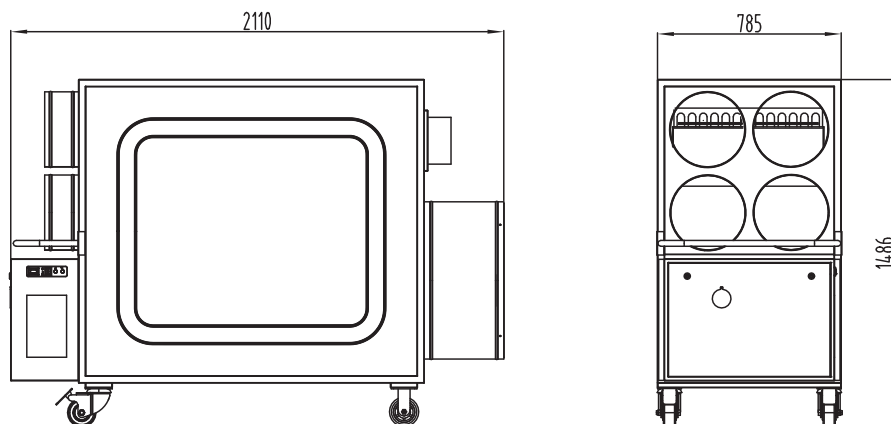
рис. 2 Размеры прибора
