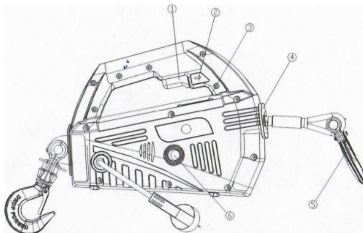
Рисунок 3. Лебедка TOR SQ-03 с ручным управлением.
