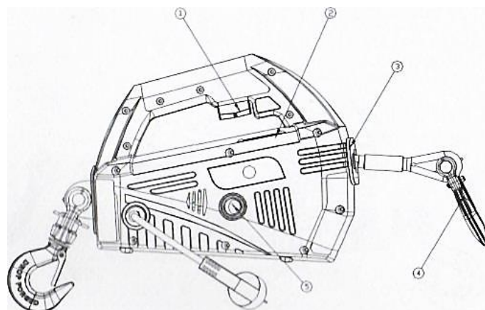
Рисунок 4. Лебедка TOR SQ-04 с дистанционным управлением.
