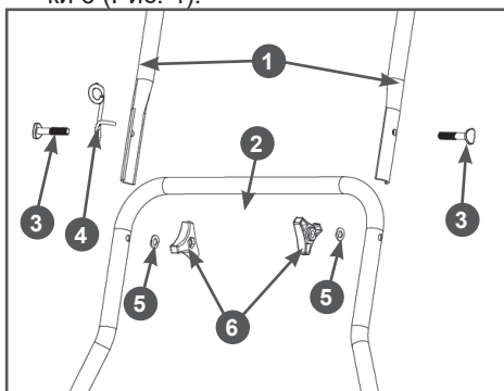
Рис. 4. Установка верхней части рукоятки
