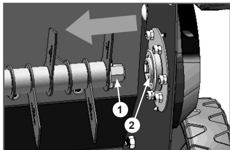
Рис. 28. Снятие рабочего валика
