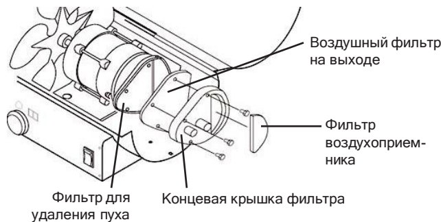
Рисунок 13. Замена фильтра
