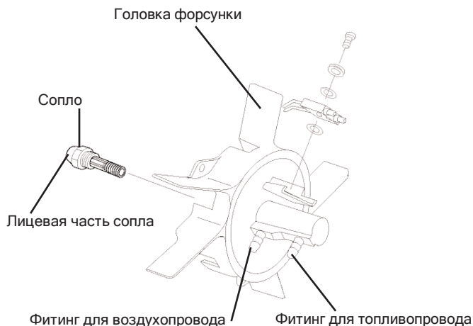
Рисунок 15. Замена сопла
