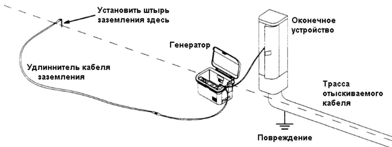
Правильное размещение штыря заземления
