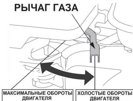
Рис. 16. Положения рычага газа
