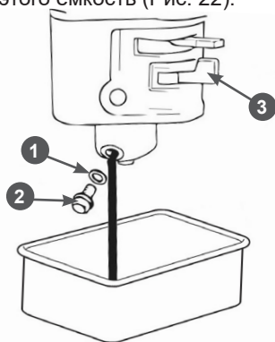
Рис. 22. Обслуживание карбюратора
