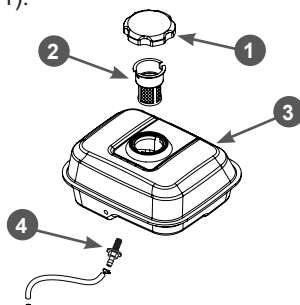
Рис. 21. Топливный бак и топливные фильтры
