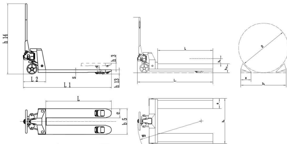
Рис. 2: Технические характеристики
