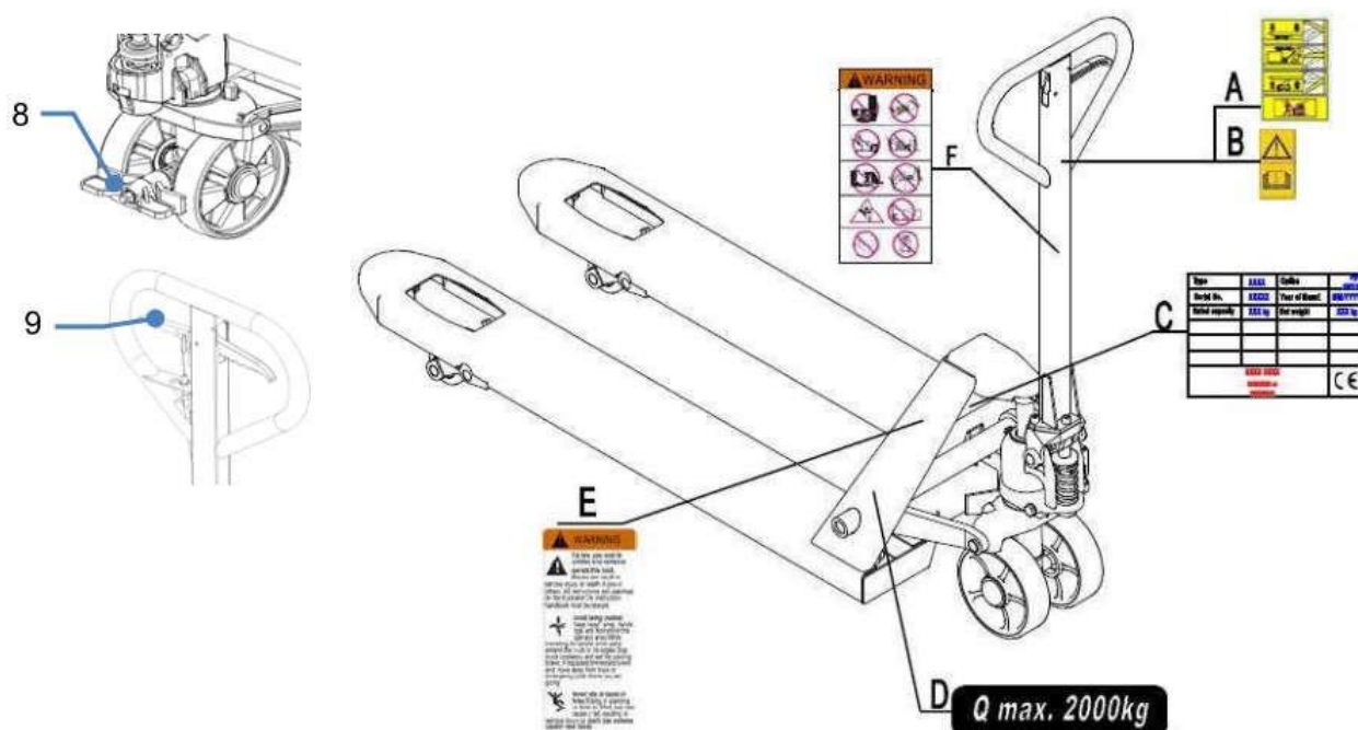
Рис. 3: Предупреждающие надписи
