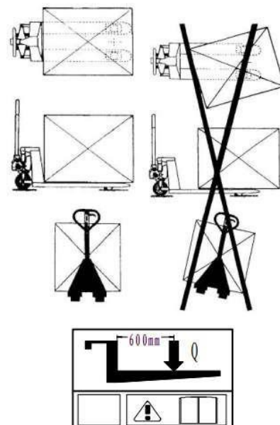
Рис. 10: Размещение груза
