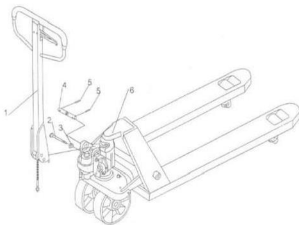
Рис. 5: Монтаж ручки
